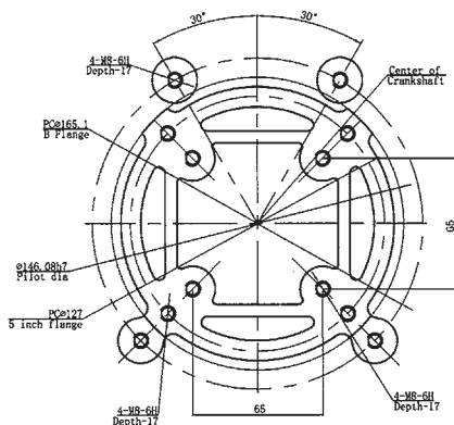
Flangia Flange Mod. K1 - G1
