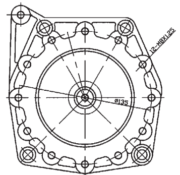
Flangia Flange Mod. G4
