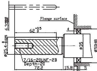
Albero Shaft Mod. K1
